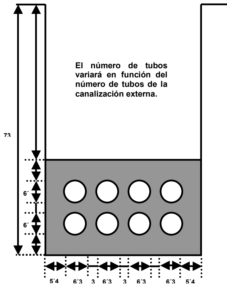
APÉNDICE 4: EJEMPLO DE SECCIÓN TRANSVERSAL DE CANALIZACIÓN DE ENLACE SUBTERRÁNEA DE 8 TUBOS.
